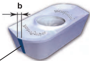
Зачищающая режущая кромка для фрезерования плоскостей
